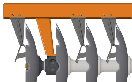
Posição limpadores no chassi traseiro
