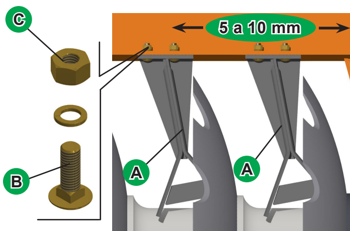
Posição limpadores no chassi traseiro
